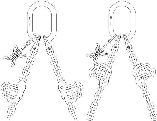
Abb. 6: Mehrstrang-Montage
