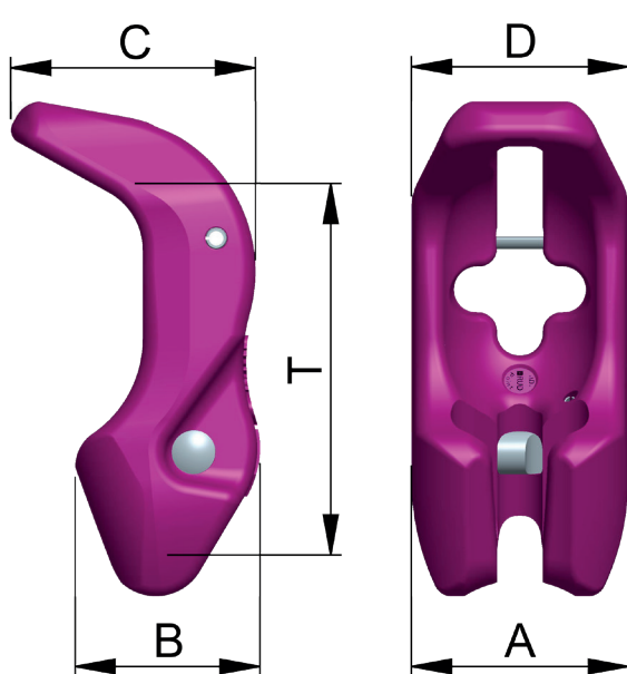
Abb. 29: Bemaßung IMVK/VMVK/BSEK
