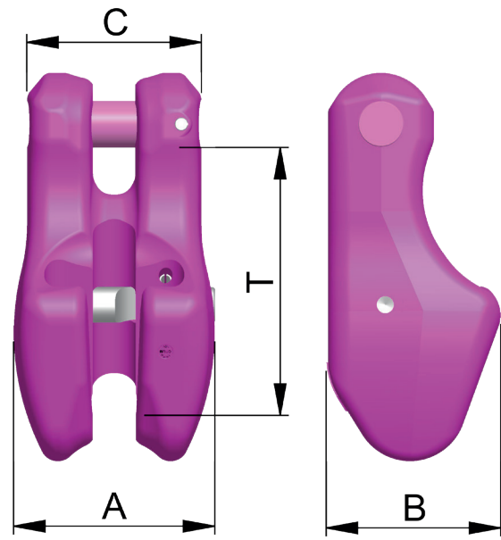
Abb. 30: Bemaßung VV
