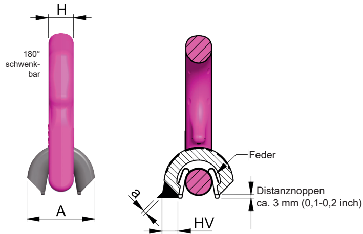
Abb. 4: Schweißnahtanordnung
