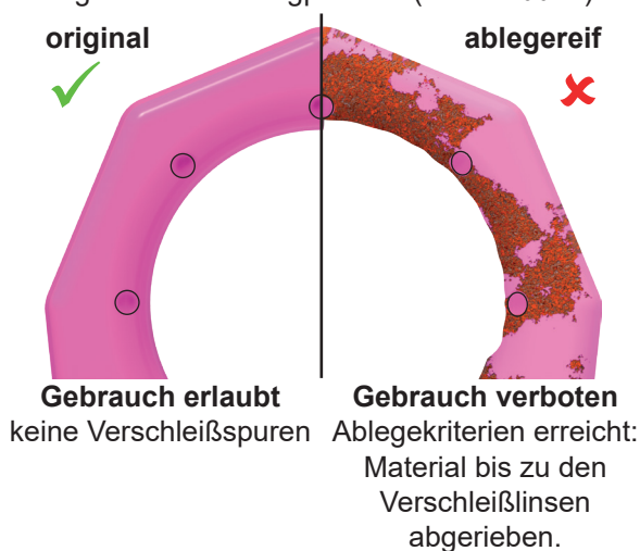
Abb. 2: Verschleißmarkierungen
