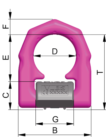
Abb. 3: Bemessung
