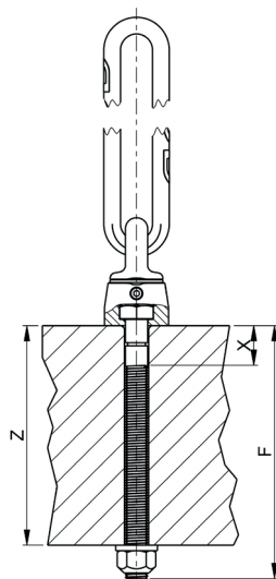
Abb. 16: Gewindelänge Fvario
