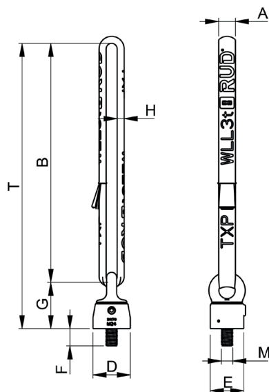
Abb. 15: Maßbild
