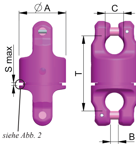
Abbildung 3: Bemaßung UW-PP/VUW-28
