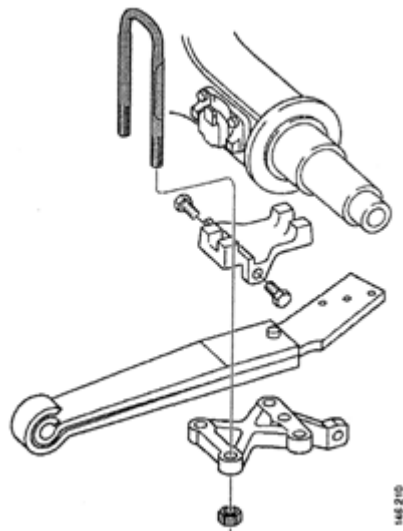
12:02-01 Luftfederung , Mechanische Teile, Arbeitsbeschreibung.
